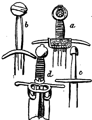
Рис. 2. Рукоятки средневековыхъ мечей западнаго издѣлья: а) мечъ св. благовѣрнаго князя Тимофея, предъ крещеніемъ именованнаго Довмонтомъ, находившійся въ Троицкомъ соборѣ, при мощахъ его, въ Псковѣ; б) мечъ XIII вѣка, на которомъ имѣется готскіи письменами надпись „Maria“; хранится въ парижскомъ артиллерійскомъ музеѣ; в) мечъ XI вѣка изъ San Agata dei Goti въ неаполитанской области; хранится въ музеѣ г. Эрбаха, д) мечъ съ т. наз. „ ras d'âne “ XV вѣка.
