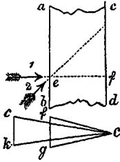
Рис. 5. Чертежъ, разъясняющій преимущество сабли. какъ рѣзущаго орудія, а b c d есть элементъ клинка меча, въ которомъ ab — лезвіе, cd — тылье. Если предметъ, который долженъ быть разрѣзанъ мечемъ, приходится въ перпендикулярномъ положеніи къ лезвію, какъ показываетъ стрѣлка № 1, то поперечное сѣченіе клинка, которымъ наносится ударъ, по линіи ef представится въ видѣ треугольника f g c; если же предметъ приходится въ косвенномъ положеніи къ лезвію, какъ показываетъ стрѣлка № 2, то поперечное сѣченіе клинка представится въ видѣ треугольника e k c, — уголъ котораго (на c) будетъ значительно острѣе и, следовательно, при одинаковыхъ условіяхъ, рѣзущая сила больше. Для достиженія этой большей остроты угла, въ некоторыхъ странахъ Востока употребляютъ такой прѣмъ, что ударяютъ мечемъ косвенно, стараясь, чтобы въ моментъ удара онъ не только расклевало, но и разрывало (дергая его къ себѣ). Но тотъ же результатъ получается при употребленіи клинка вездѣ (придаемъ ему форму сабли), потому что тогда, и при обыкновенно разрывающемъ ударѣ, лезвіе будетъ падать на предметъ косвенно.
